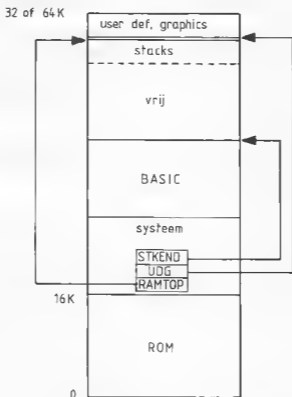
Afb. 1-1 Geheugenindeling na aanschakelen
